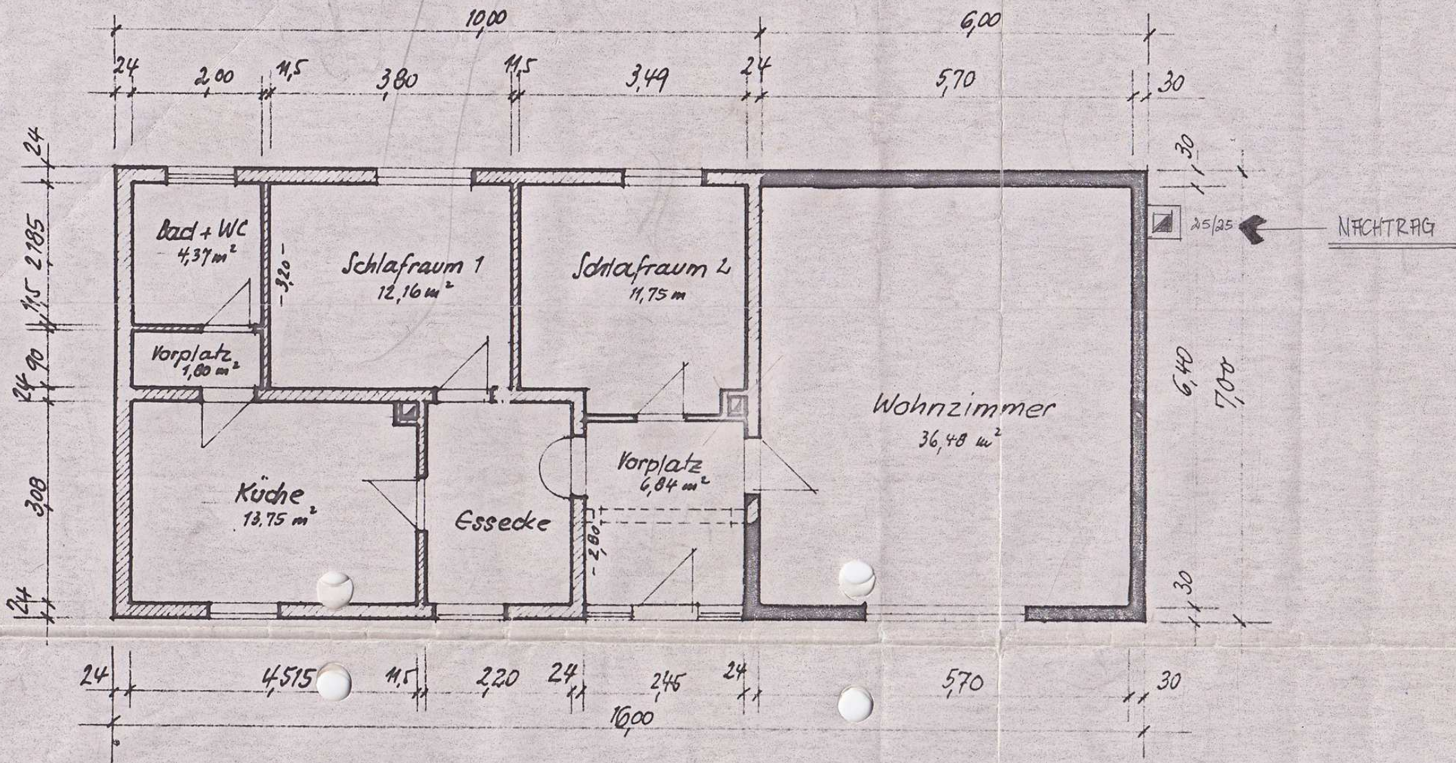
- Erdgeschoßgrundriß -
